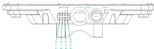
· Панель ввода/вывода уличного блока ·
